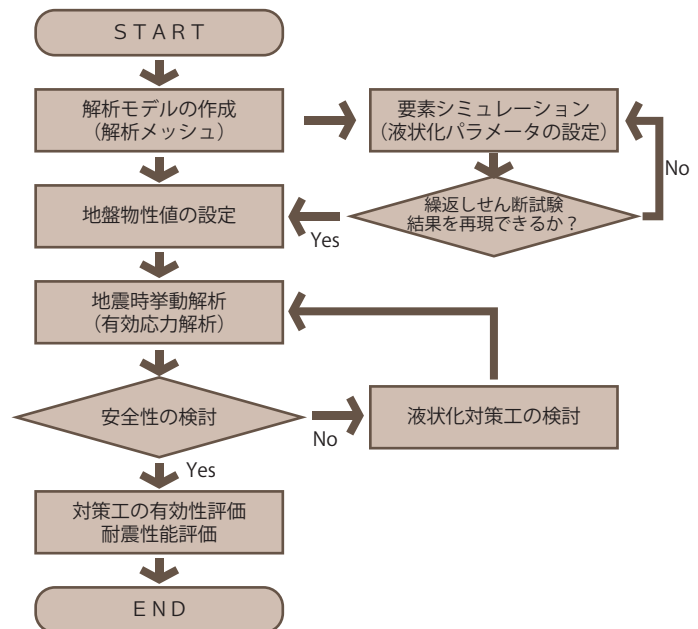
有効応力解析検討フロー図
