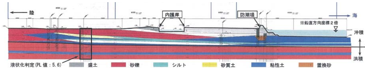
図-1 地質断面
