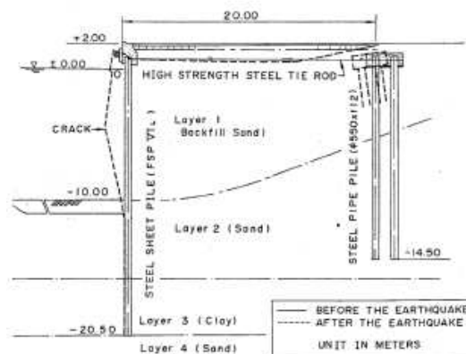
図-1 被災状況
