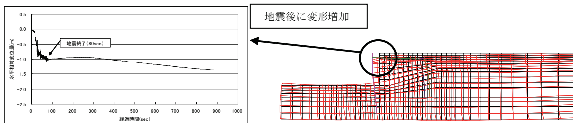
図-5 矢板の水平変位
