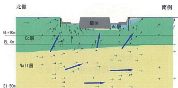
図7 流向図(断面)
