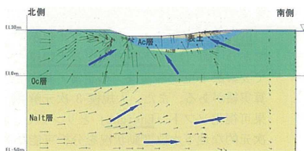
図5 流向図(断面)
