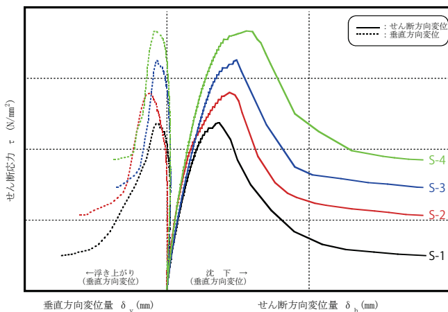
岩盤せん断試験結果例
