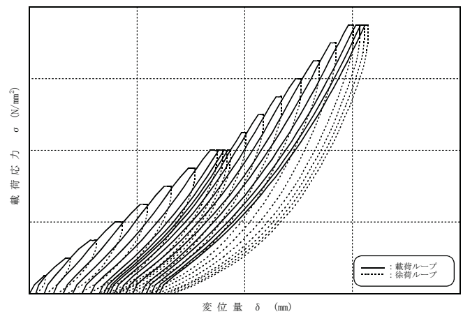
岩盤変形試験結果例
