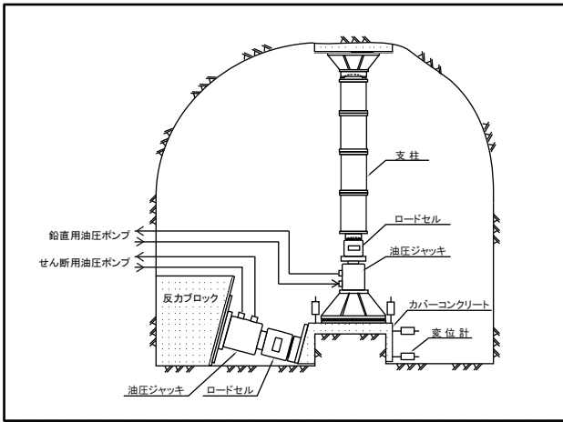
岩盤せん断試験装置概要図
