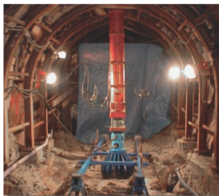
岩盤変形試験
