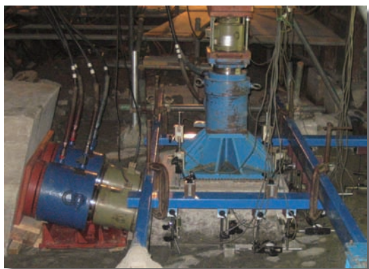
岩盤せん断試験
