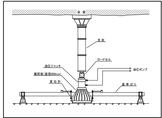
岩盤変形試験装置概要図
